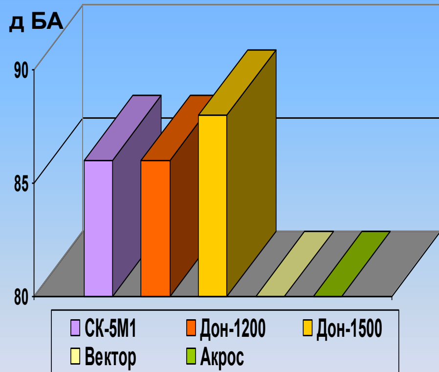
Зерноуборочные комбайны
