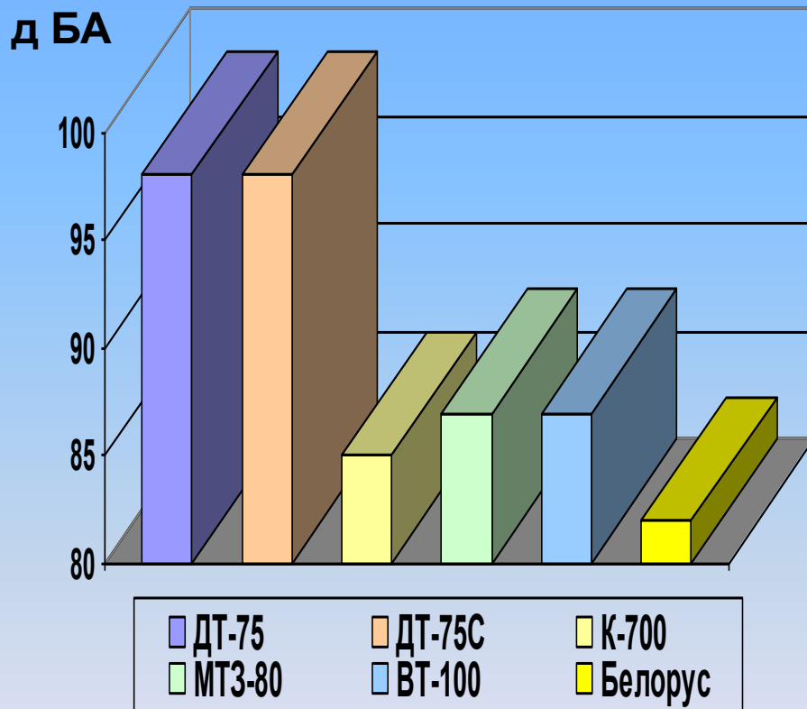
Тракторы
